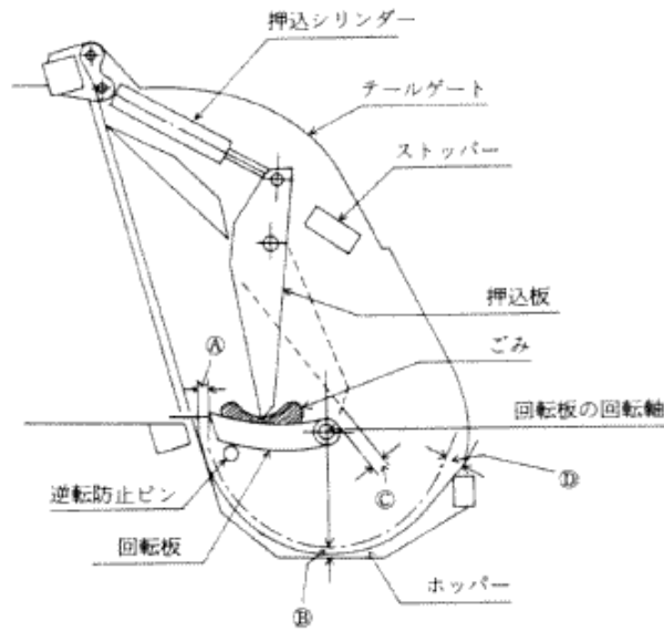
第1図 回転式ゴミ収集車のテールゲートの構造の例
