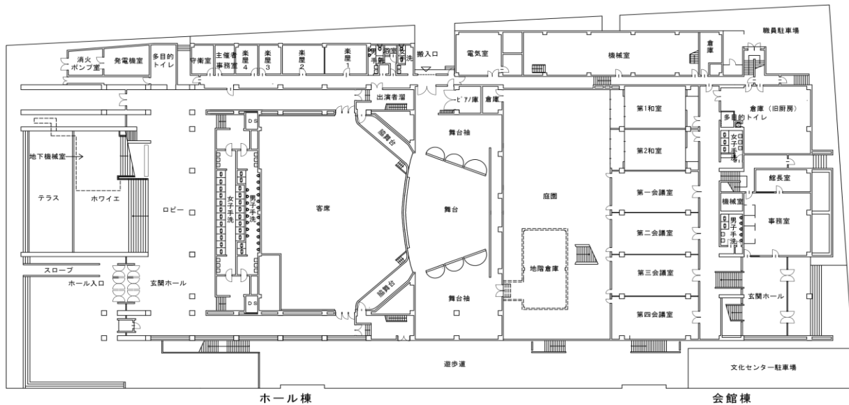
1階 平面図
