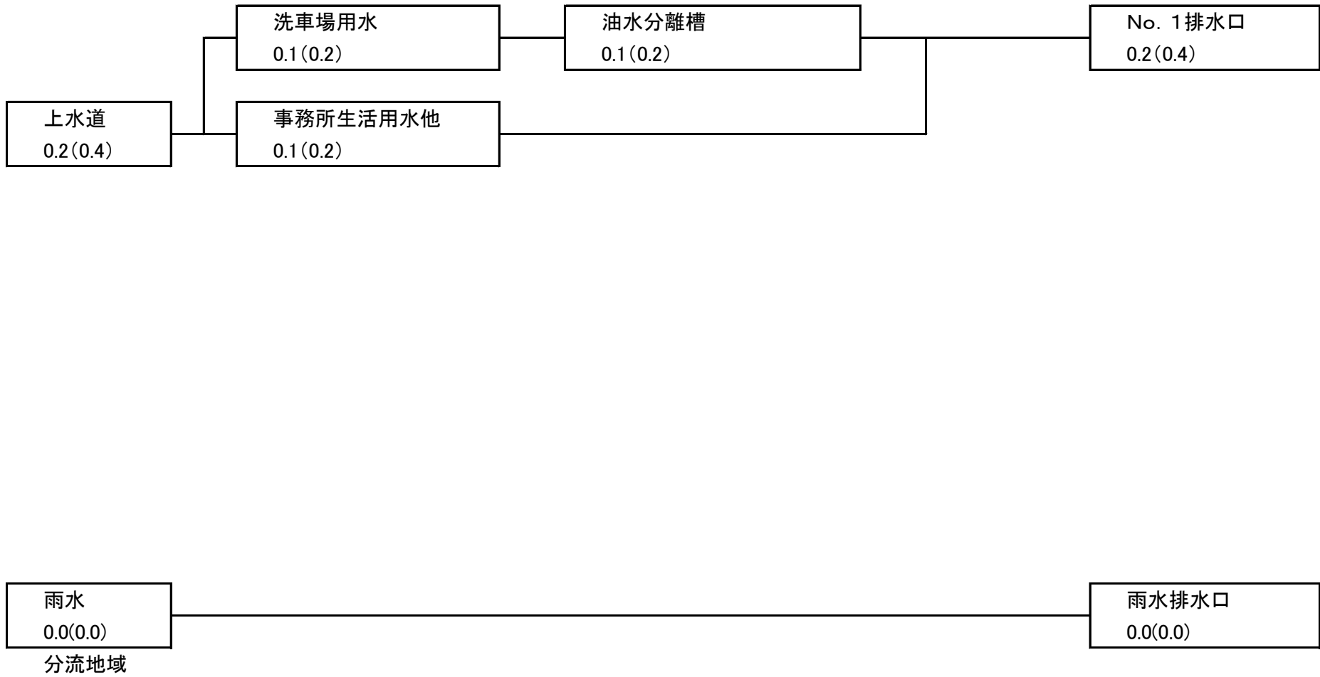
株式会社〇〇 / 排水系統図 (平均(最大) 単位:m 3 /日)
