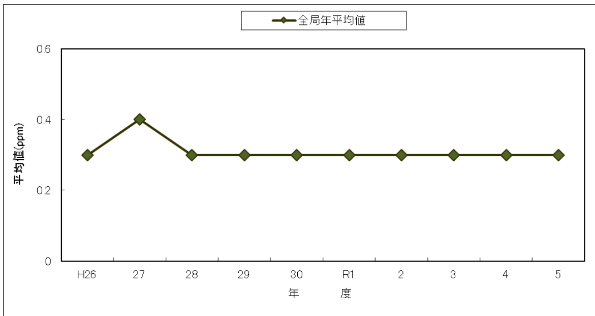
図 3-16 全局CO濃度年平均値の経年変化
