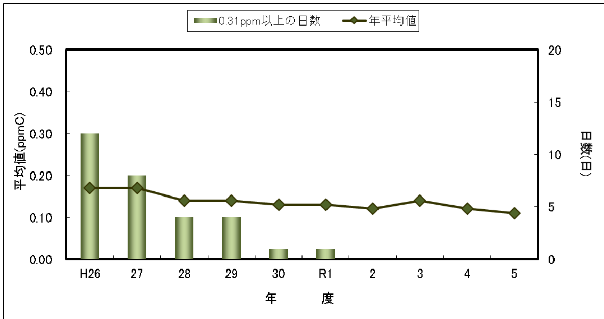
図 3-18 駅前局NMHC6-9時の3時間平均値の年平均値と0.31ppmC超過日数の経年変化
