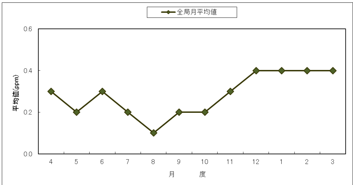
図 3-17 全局CO濃度月平均値の経月変化
