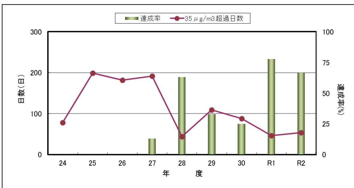
図2-12 一般環境大気測定局PM2.5環境基準達成率とPM2.5濃度 35\mu\text{g}/\text{m}^3 超過日数の経年変化
