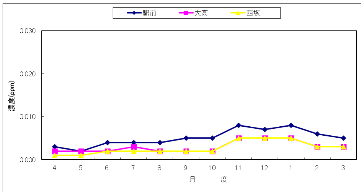
ク 一酸化窒素濃度の経月変化（月平均値）
