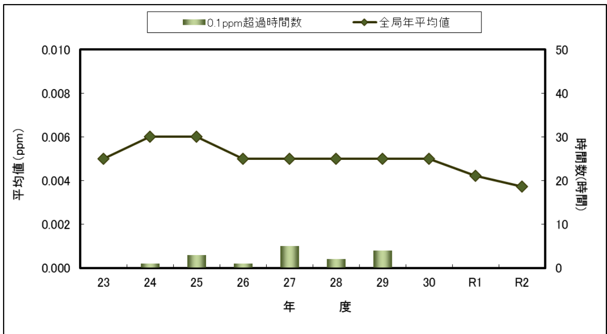
图 3-1 全局SO 2 濃度年平均値の経年変化
