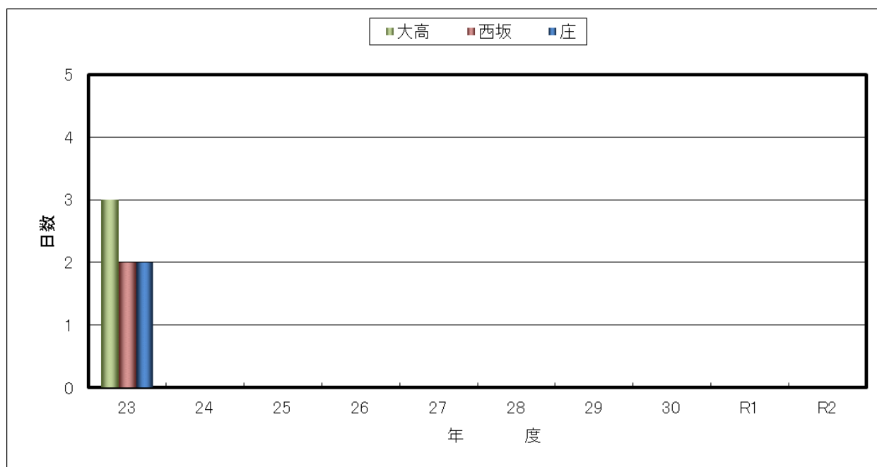
ス 浮遊粒子状物質濃度の日平均値が 0.1\text{mg}/\text{m}^3 を超えた日数の経年変化
