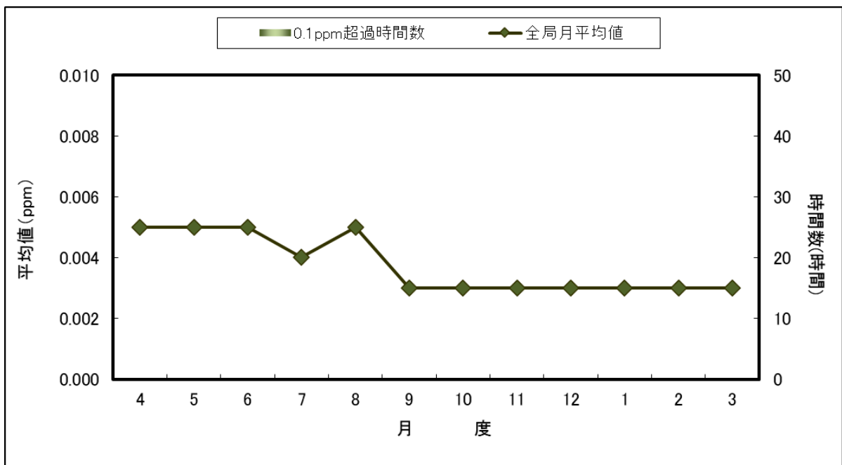
图 3-2 全局SO 2 濃度月平均値の経月変化
