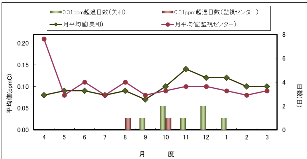
図 3-10 NMHC6-9時の3時間濃度の月平均値と0.31ppmC超過日数の経月変化
