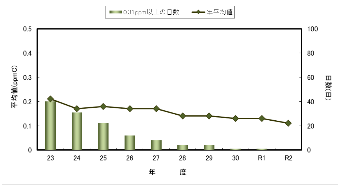
図 3-18 駅前局NMHC6-9時の3時間値年平均濃度と0.31ppmC超過日数の経年変化
