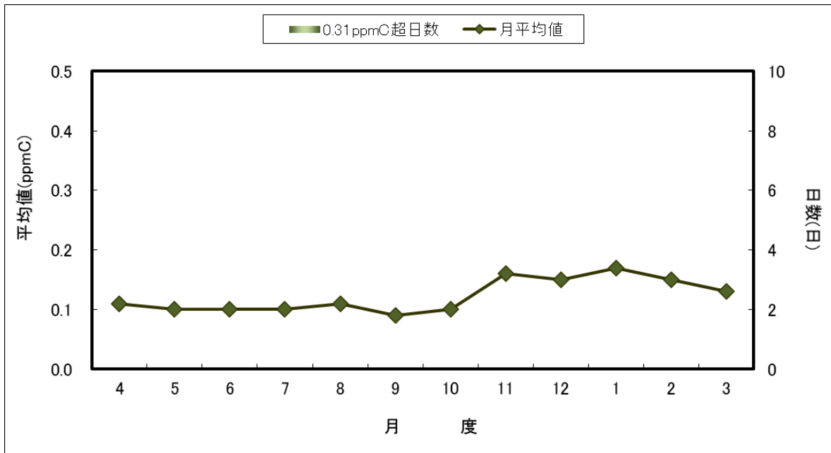
図 3-19 駅前局NMHC6-9時の3時間値月平均濃度と0.31ppmC超過日数の経月変化
