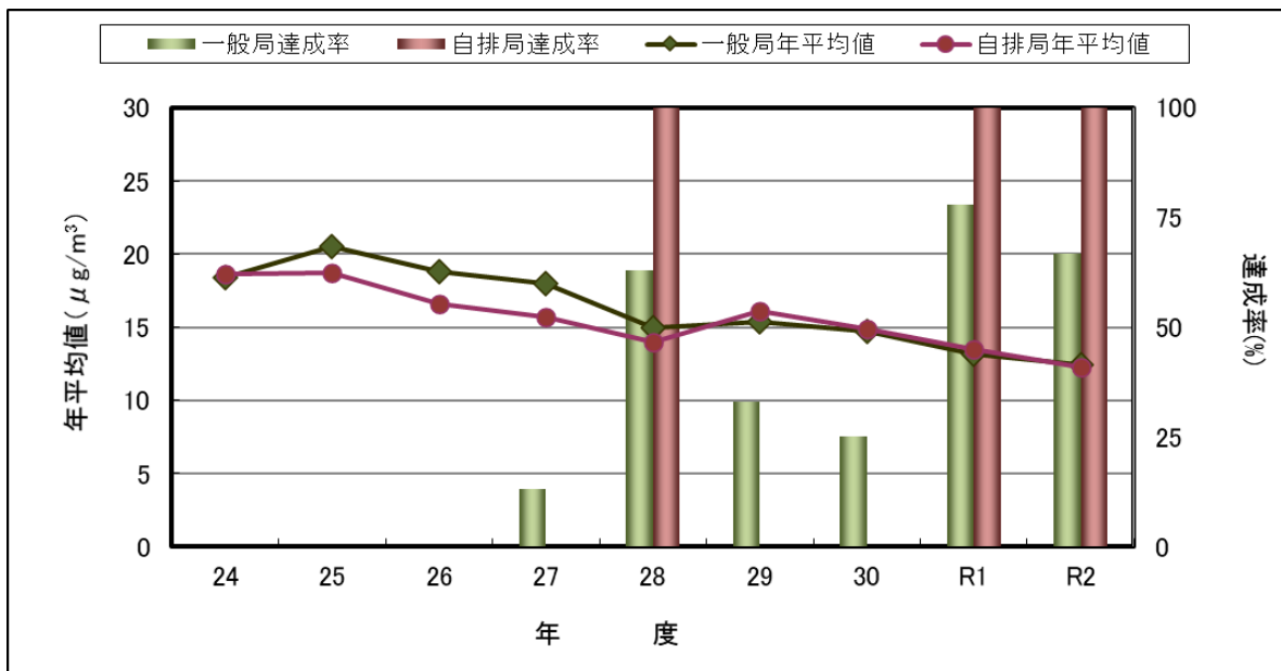
図 2-14 局種別PM2.5環境基準達成率とPM2.5濃度年平均値の経年変化
