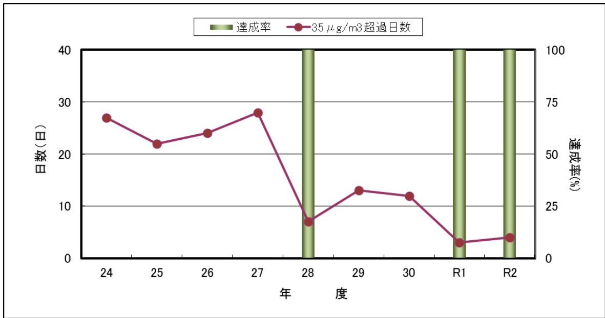
図 2-13 自動車排ガス測定局PM2.5環境基準達成率とPM2.5濃度35µg/m³超過日数の経年変化
