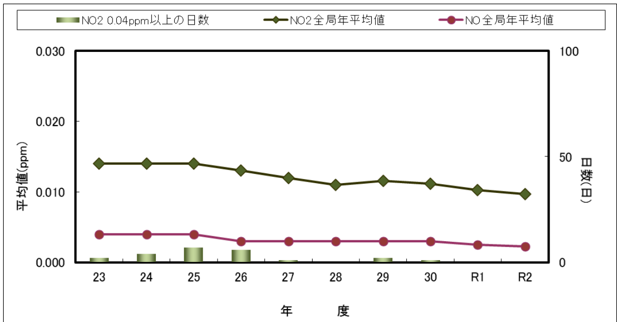
図 3-14 全局NO 2 、NO濃度年平均値とNO 2 濃度0.04ppm以上の日数の経年変化
