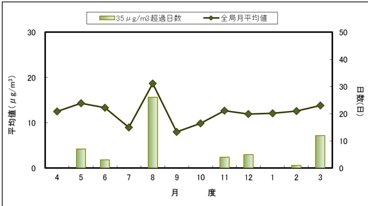
図3-13 全局PM2.5濃度月平均値と 35 \mu\text{g}/\text{m}^3 超過日数の経月変化
