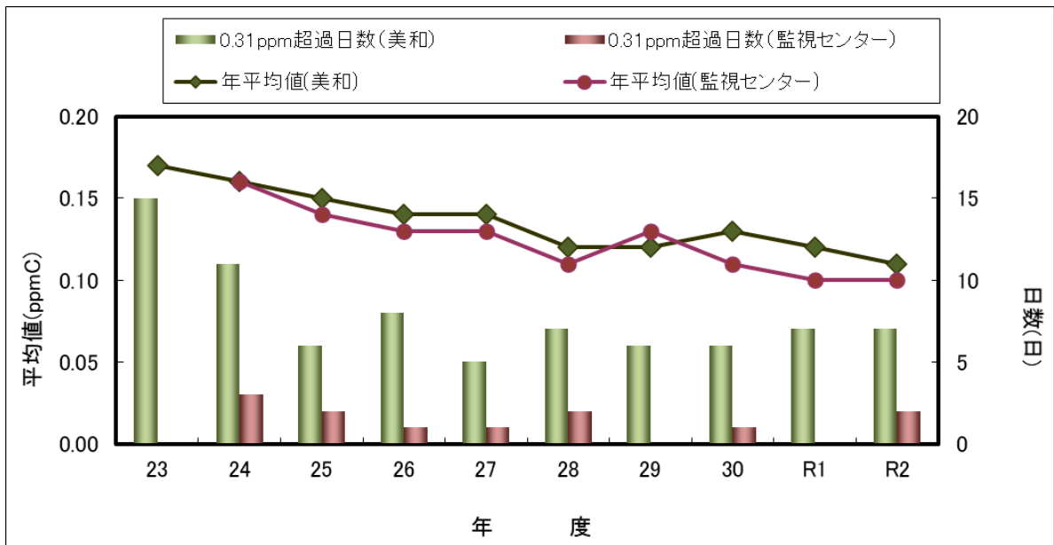
図 3-9 NMHC濃度と0.31ppmC超過日数の経年変化
