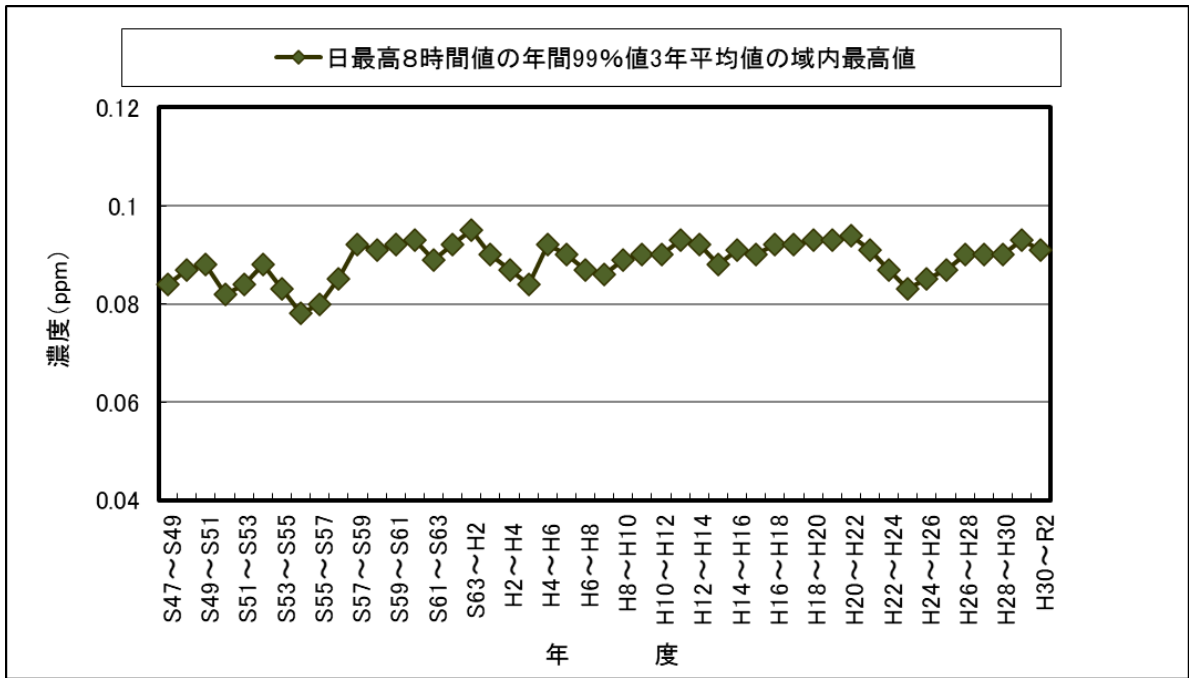
図 2-6 0x日最高8時間値の年間99%値3年平均値の域内最高値の経年変化 (※平成28年2月17日環水大大発第1602171号 光化学オキシダントの環境改善効果を適切に示すための指標に係る測定値の取り扱いについて)
