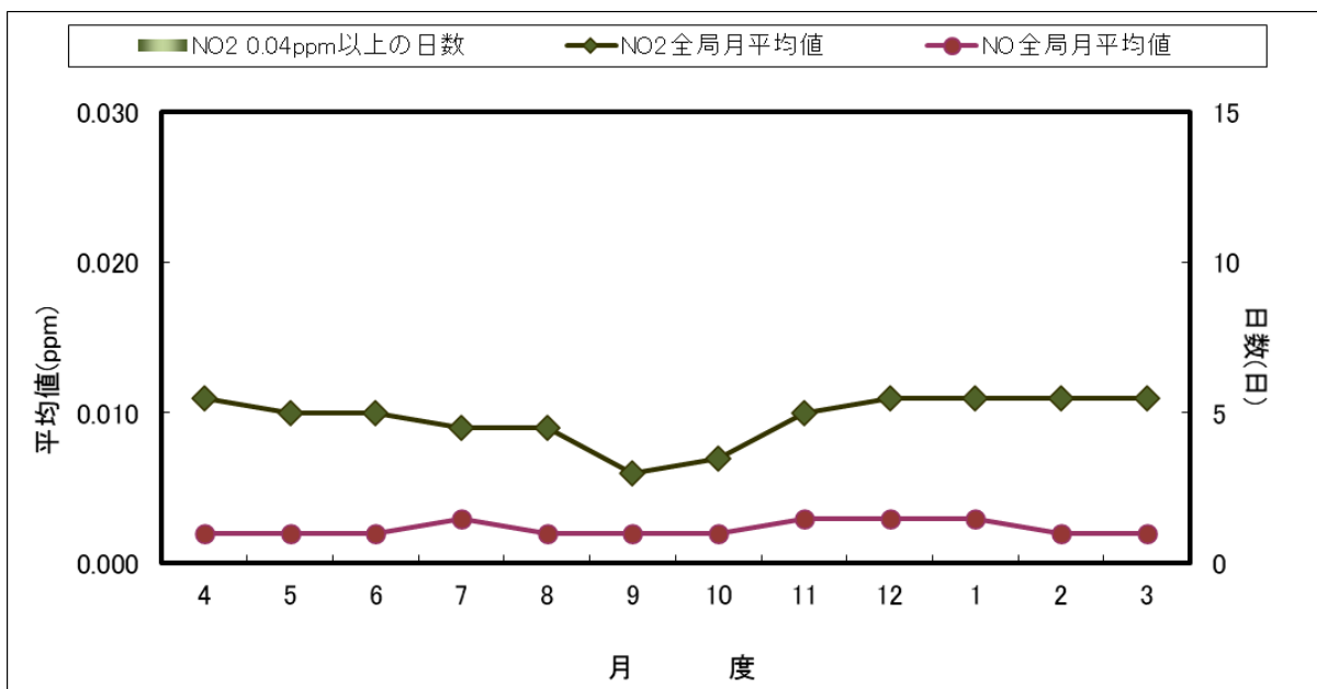
図 3-15 全局NO 2 、NO濃度月平均値とNO 2 濃度0.04ppm以上の日数の経月変化
