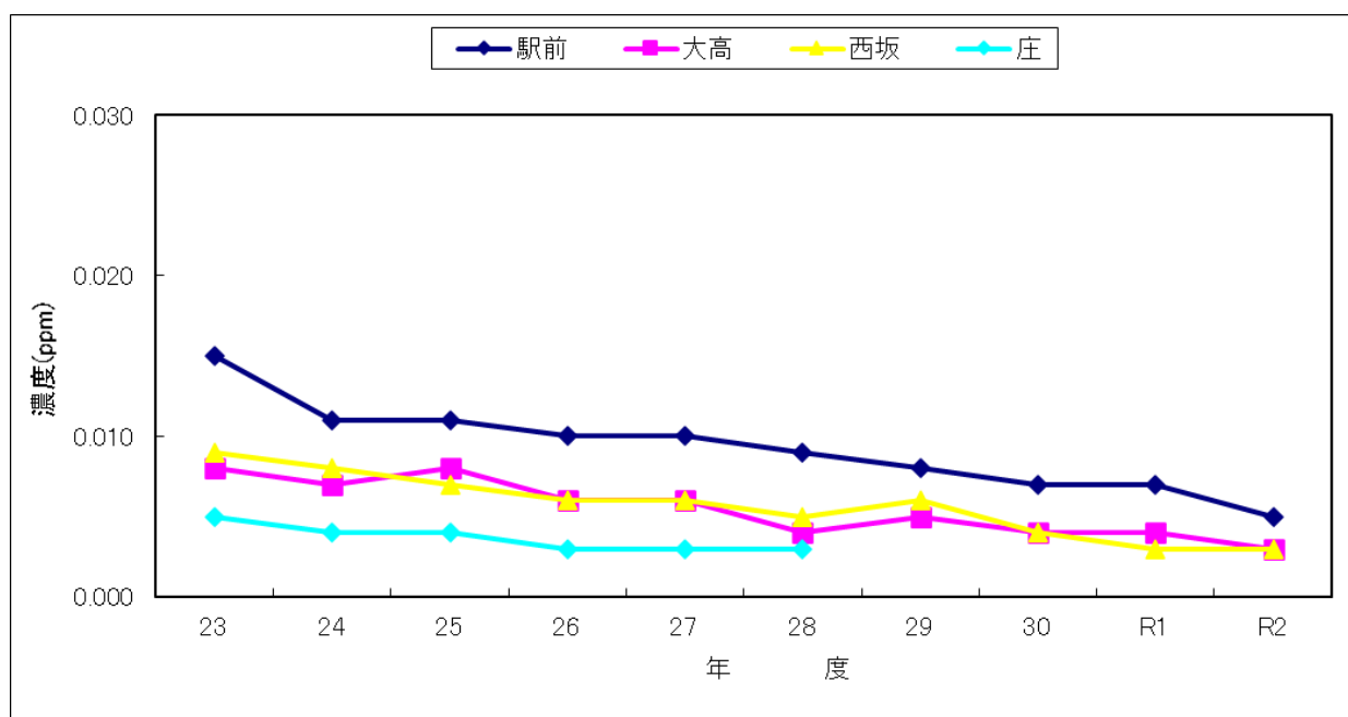
キ 一酸化窒素濃度の経年変化（年平均値）
