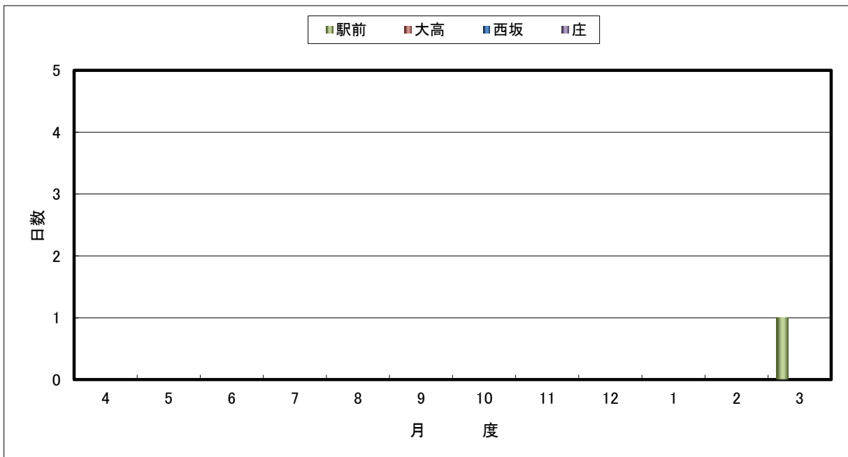
カ 二酸化窒素濃度の日平均値が0.04ppm以上となった日数の経月変化
