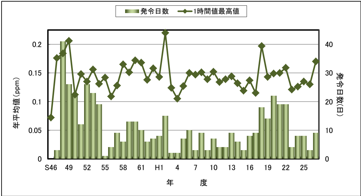
図 2-6 全局O 3 濃度 1 時間値最高値と光化学オキシダント情報等発令日数の経年変化
