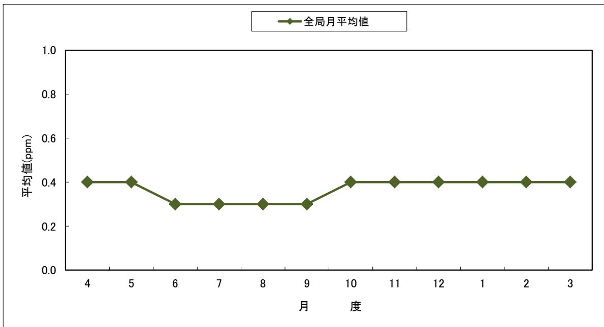
図 3-17 全局CO濃度月平均値の経月変化
