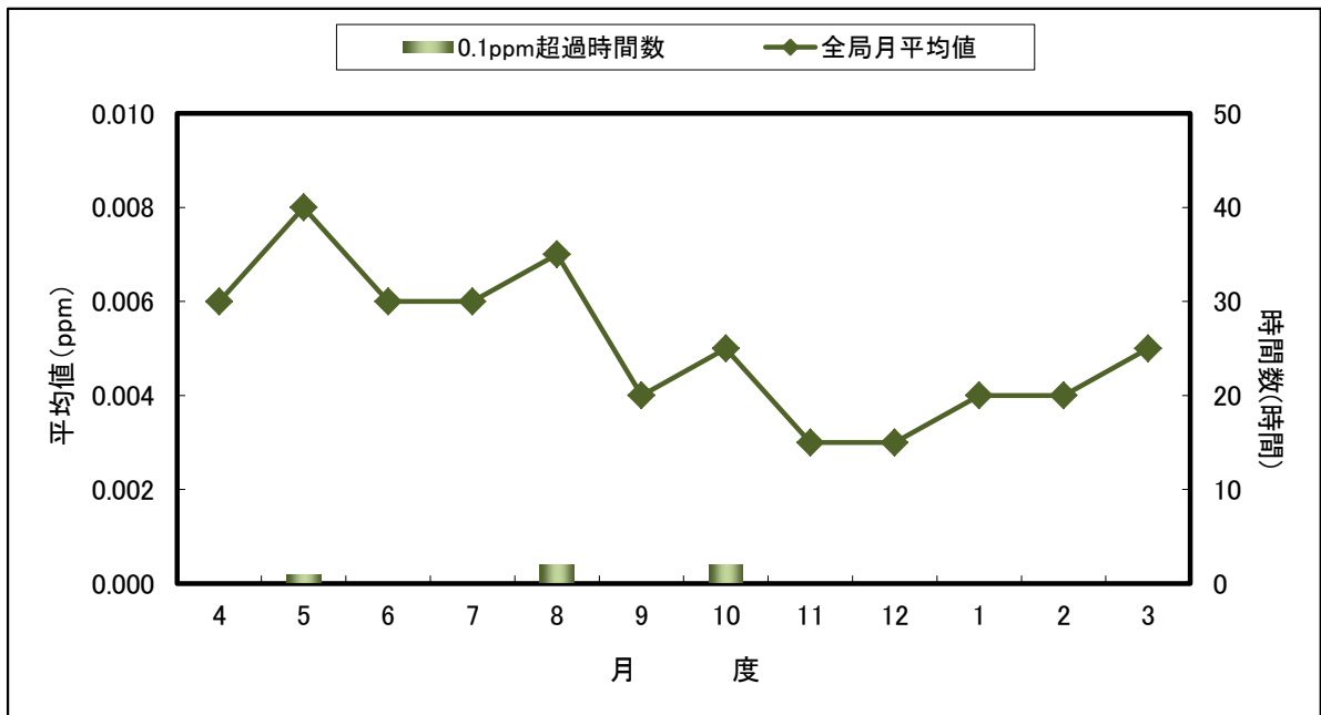
図 3-2 全局SO 2 濃度月平均値の経月変化
