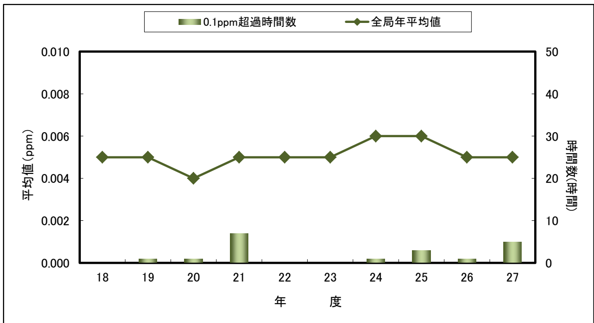
図 3-1 全局SO 2 濃度年平均値の経年変化
