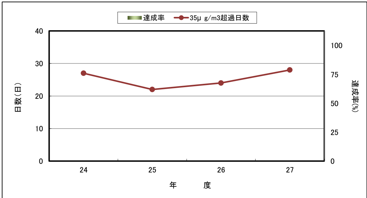
図 2-11 自動車排ガス測定局PM2.5長期的評価達成率とPM2.5濃度35 \mu g/m 3 超過日数の経年変化
