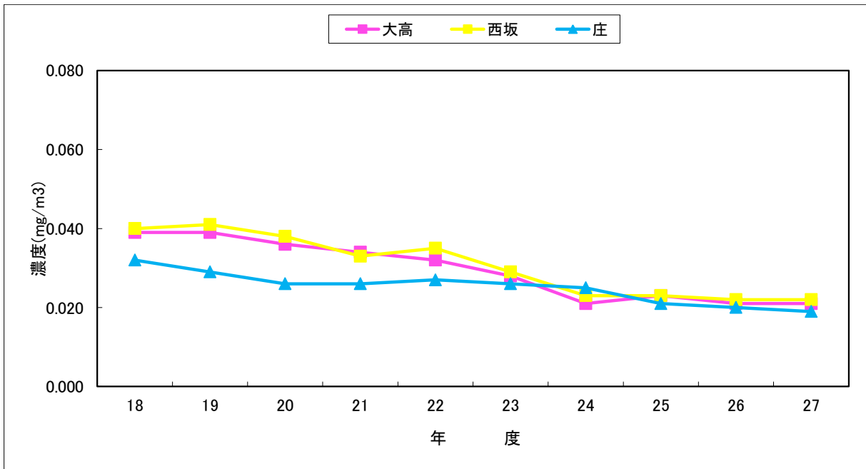
サ 浮遊粒子状物質濃度の経年変化（年平均値）
