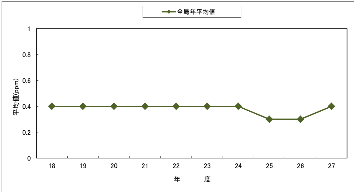
図 3-16 全局CO濃度年平均値の経年変化
