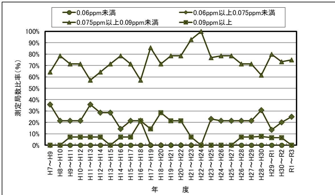
図 2-7 0x新指標の濃度別測定局数比率の経年変化
