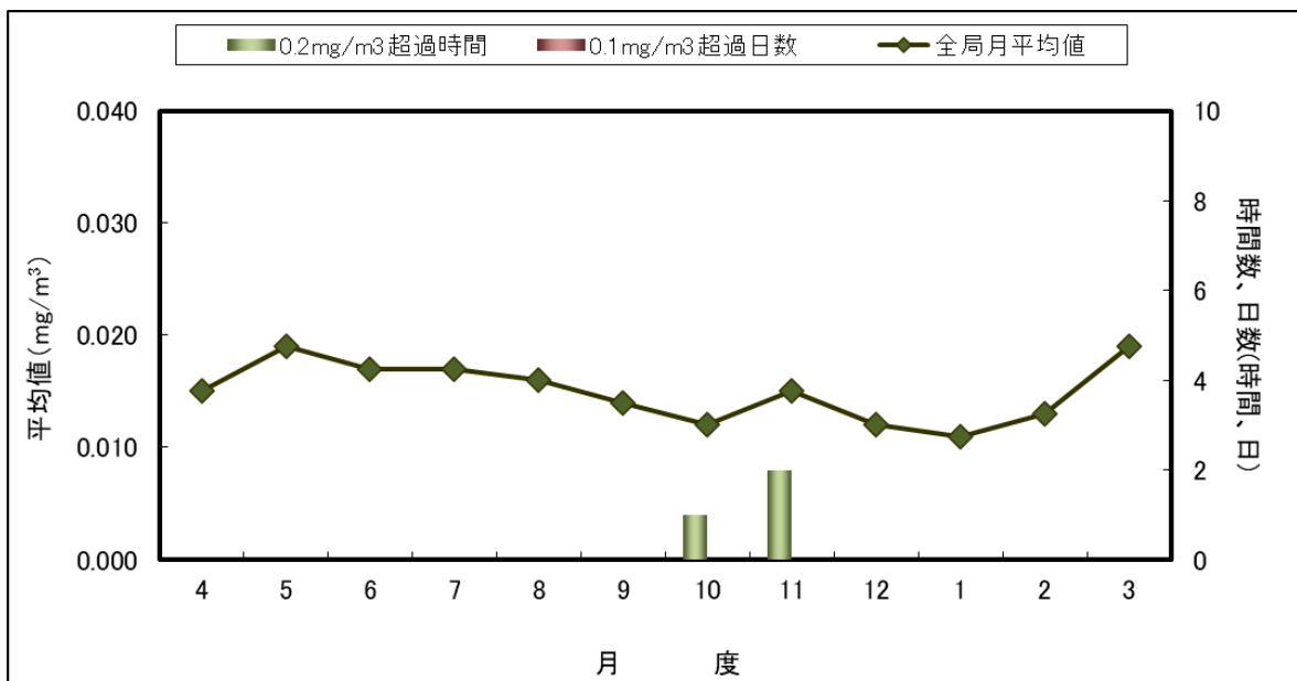
図 3-12 全局SPM濃度月平均値、0.2mg/m 3 超過時間数及び0.1mg/m 3 超過日数の経月変化
