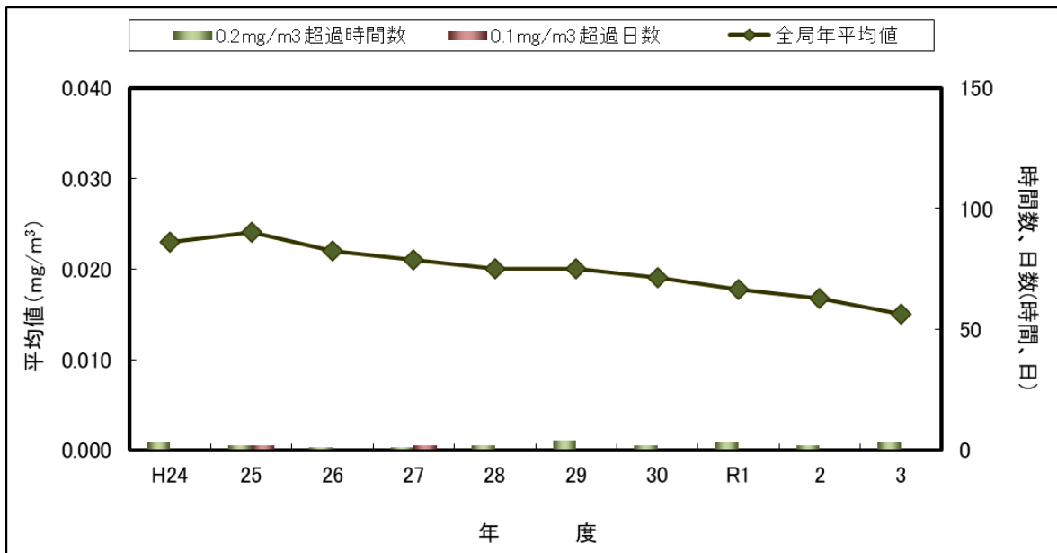
図 3-11 全局SPM濃度年平均値、0.2mg/m 3 超過時間数及び0.1mg/m 3 超過日数の経年変化
