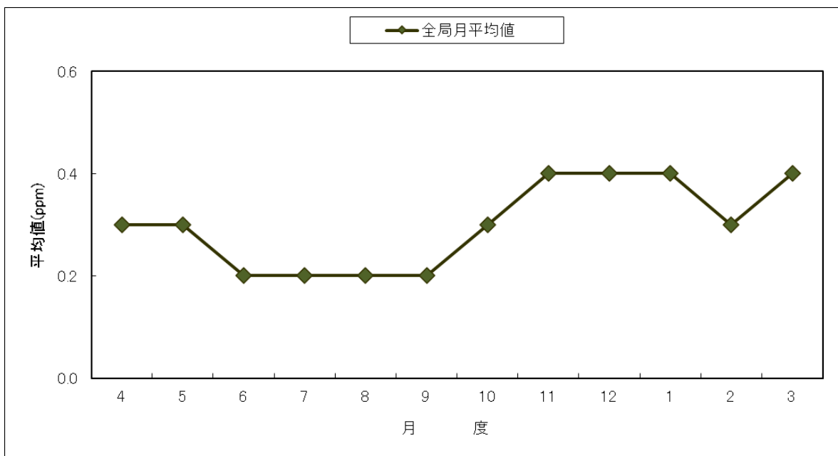
図 3-17 全局CO 2 濃度月平均値の経月変化
