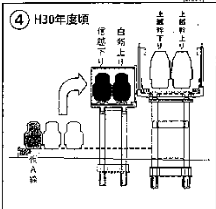
高架橋1期工事2線分が完成後、仮線を一部撤去します
