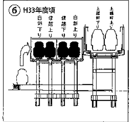
4線の高架化が完成
