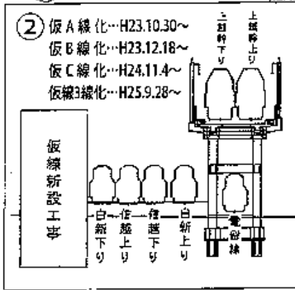
仮線を新設し、仮線完成後、新幹線側の営業線、電留線を撤去します(黄色表示:撤去する線)
