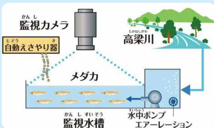
▲バイオアッセイ装置の仕組み
