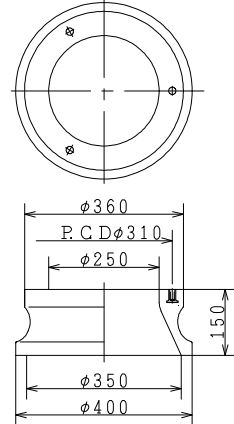
倉敷市型円形1号150CA (円形1号RB25CA)
