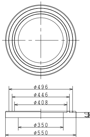
倉敷市型円形1号40P (円形1号RB25P)
