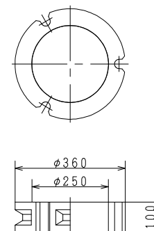
倉敷市型円形1号100K (円形1号RB25K)
