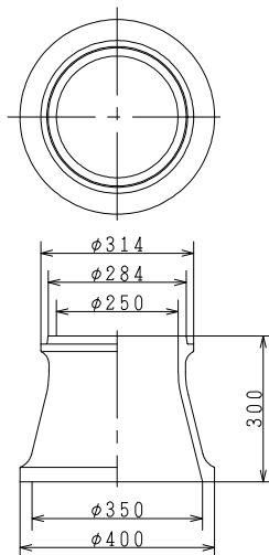
倉敷市型円形1号300C (円形1号RB25C)
