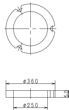
倉敷市型円形1号50K (円形1号RB25K)
