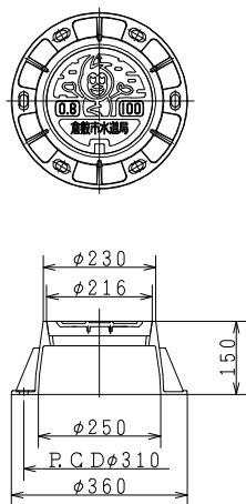
倉敷市型円形1号鉄蓋 (円形1号(250))
