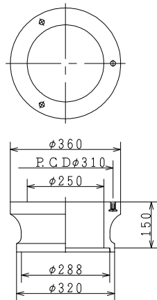
倉敷市型円形1号150A (円形1号RB25A)
