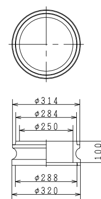
倉敷市型円形1号100B (円形1号RB25B)
