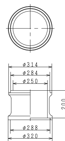
倉敷市型円形1号200B (円形1号RB25B)
