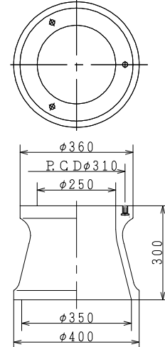
倉敷市型円形1号50K (円形1号RB25K)
