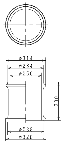
倉敷市型円形1号300B (円形1号RB25B)
