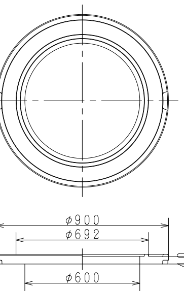
倉敷市型円形5号40P (円形5号RB70(P))
