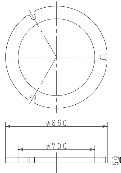
倉敷市型円形5号50K (円形5号RB50(K))
