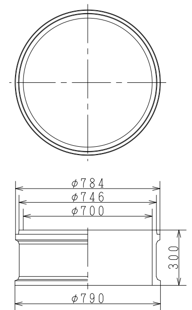
倉敷市型円形5号300C (円形5号RB70(C))
