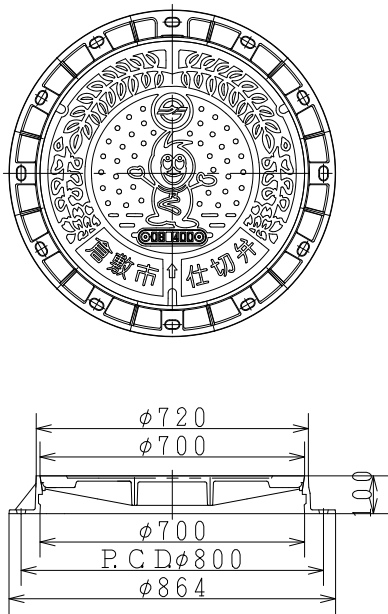
倉敷市型円形5号鉄蓋 (円形5号(700))
