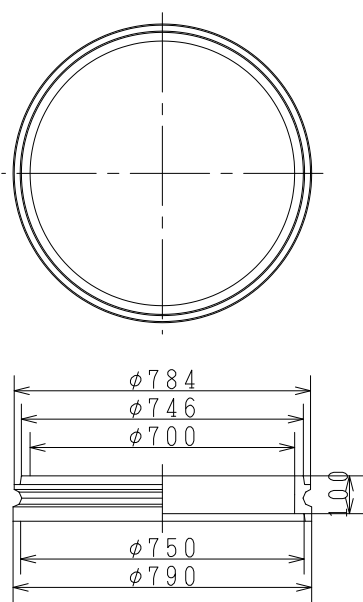
倉敷市型円形5号100B (円形5号RB70(B))
