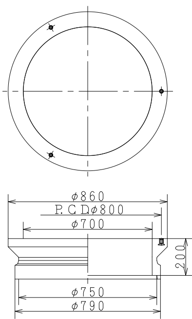
倉敷市型円形5号300C (円形5号RB70(C))
