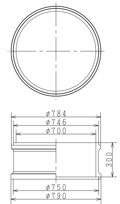
倉敷市型円形5号300B (円形5号RB70(B))
