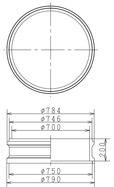
倉敷市型円形5号200B (円形5号RB70(B))
