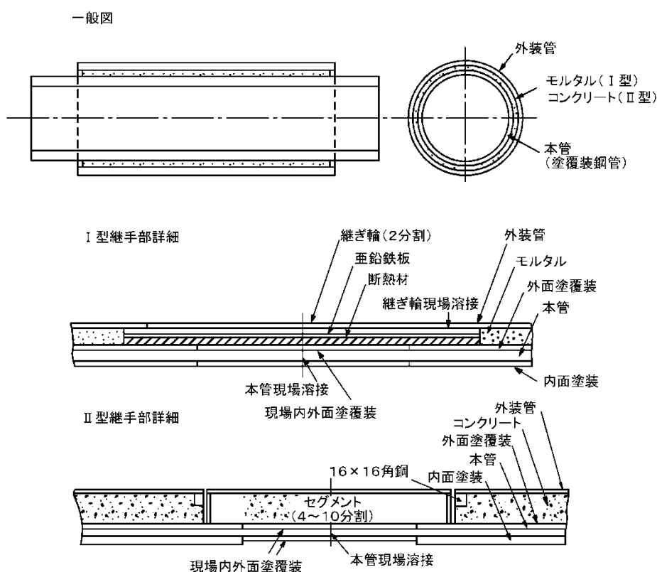
図 2－17 水道用推進鋼管
