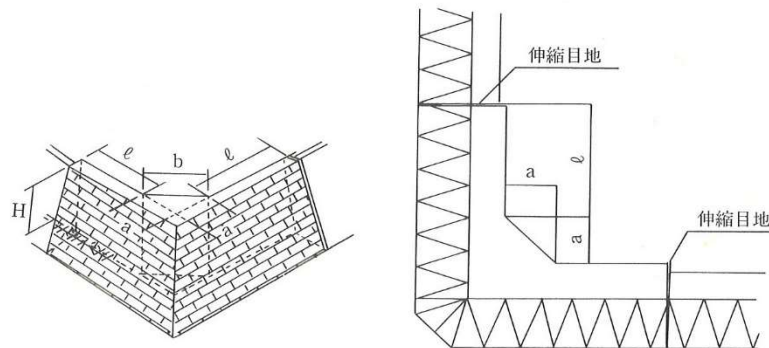
(a) 立体図
