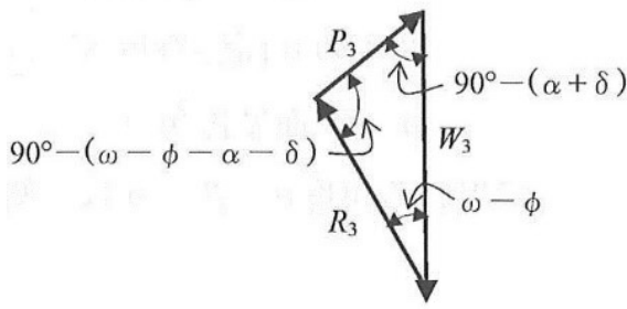
(c) 連力図
