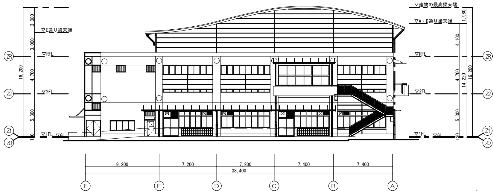
南 立面図
