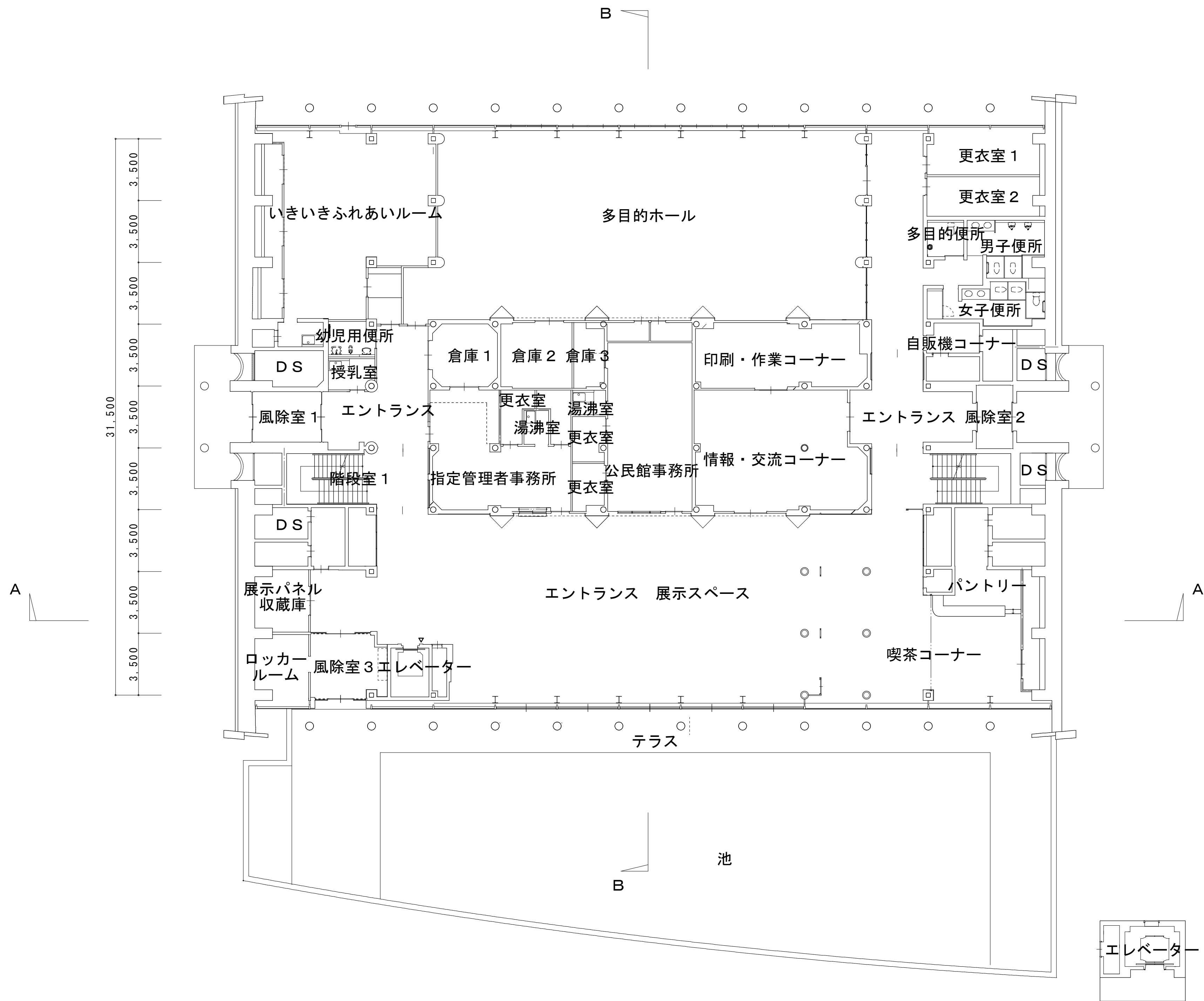
1階 平面図
