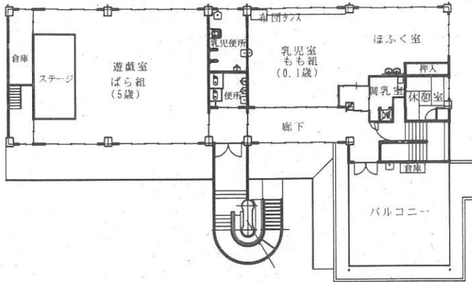
2階平面図
